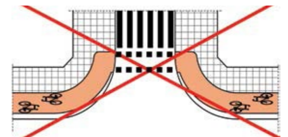
Rysunek 22 Niedopuszczalne odgięcie drogi dla rowerów przed samym przejazdem
