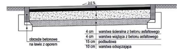
Rysunek 8 Konstrukcja drogi dla rowerów
