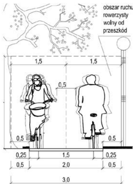
Rysunek 5 Skrajnia dla ruchu rowerowego
