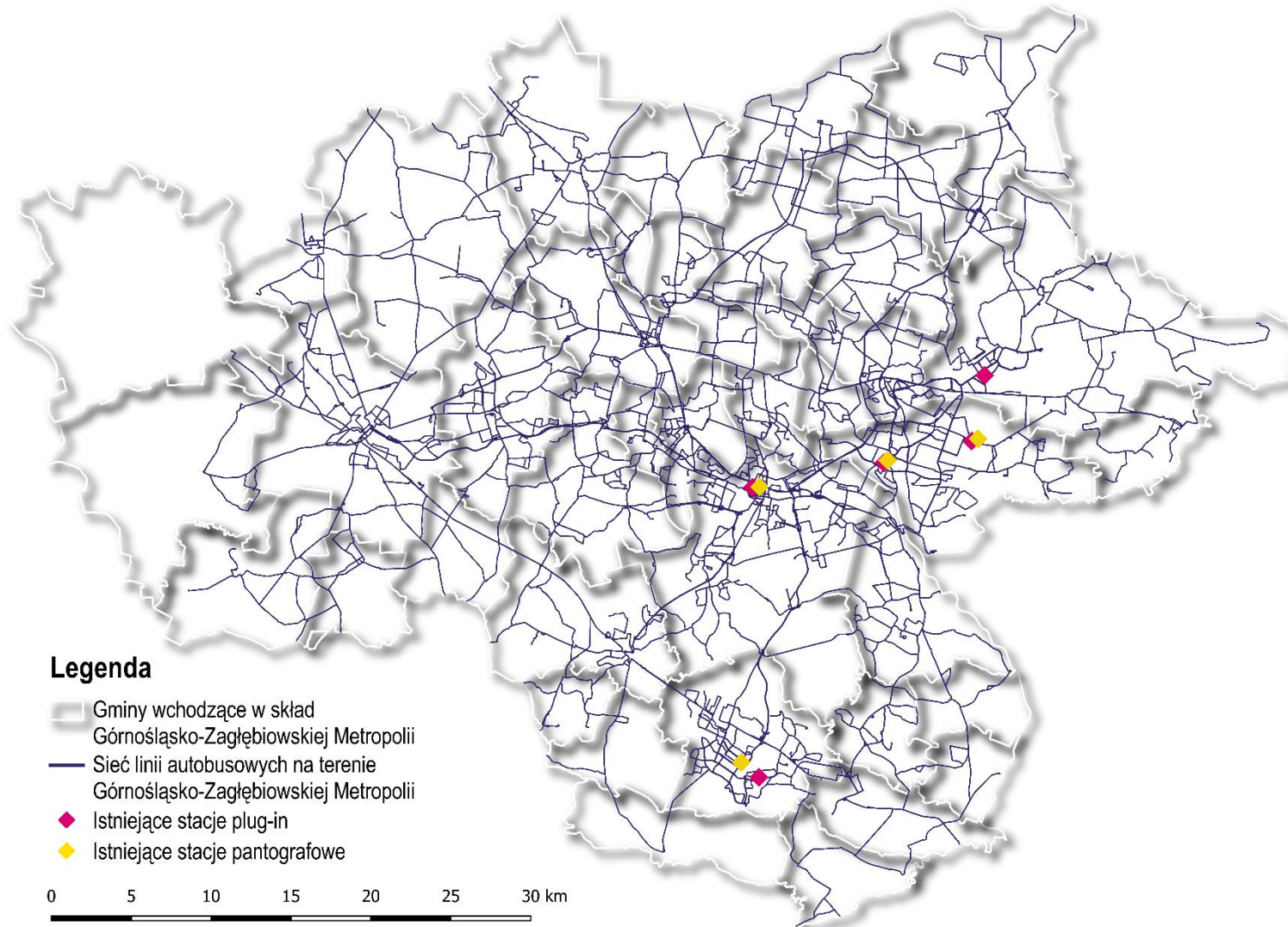
Rysunek 14. Istniejąca sieć infrastruktury do ładowania autobusów elektrycznych na obszarze Górnośląsko-Zagłębiowskiej Metropolii
