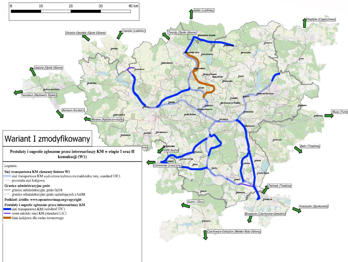
Rys. 12.3. Sieć transportowa Kolei Metropolitalnej – wariant W1A, propozycje interesariuszy KM Źródło: Suplement do dokumentu pn. Koncepcja Kolei Metropolitalnej dla Górnoszląsko-Zagłębiowski Metropolitan z wykorzystaniem metod inżynierii systemów, Katowice 2019
