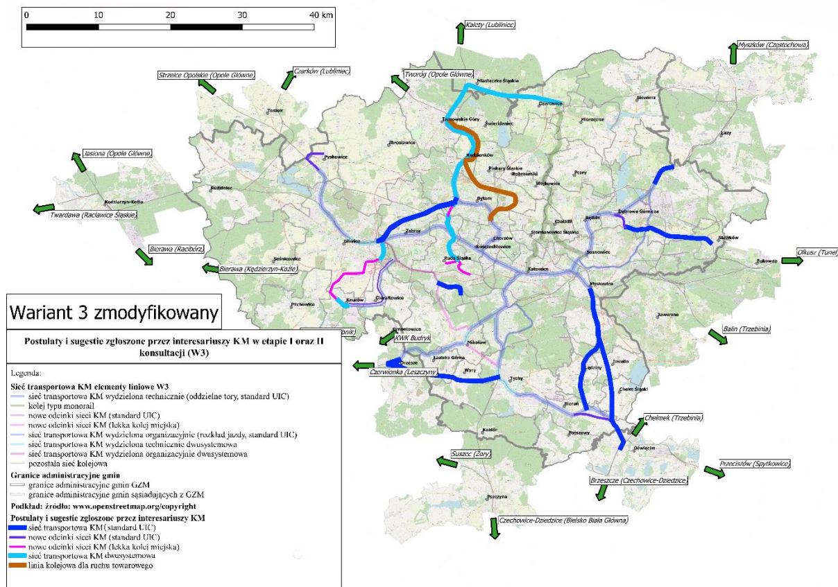
Rys. 12.7. Sieć transportowa Kolei Metropolitalnej – wariant W3A, propozycje interesariuszy Źródło: Suplement do dokumentu pn. Koncepcja Kolei Metropolitalnej dla Górnosląsko-Zagłębiowski Metropolii z wykorzystaniem metod inżynierii systemów, Katowice 2019
