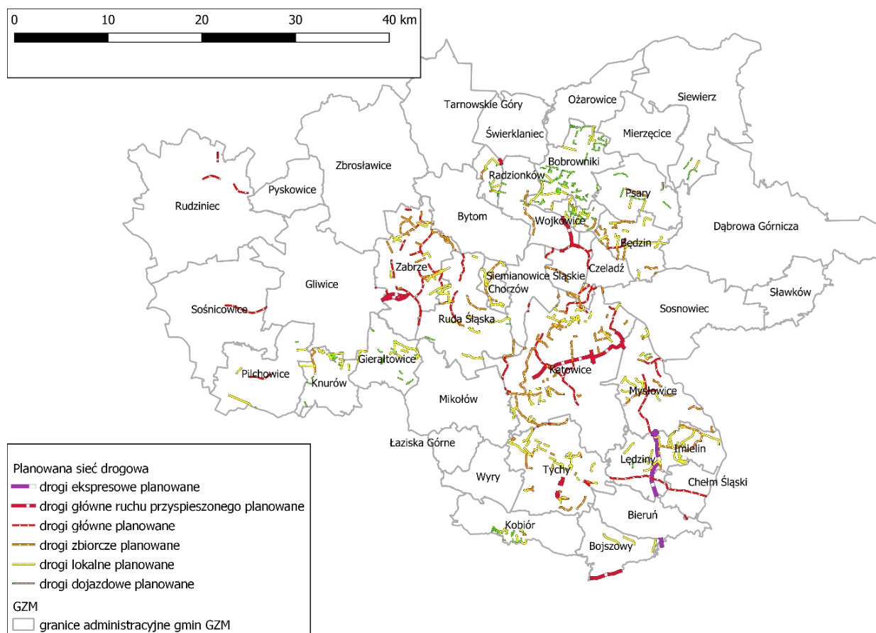
Rys. 3.13. Planowane (uwzględniające remonty) odcinki sieci drogowo-ulicznej z podziałem na klasy techniczne na obszarze GZM
