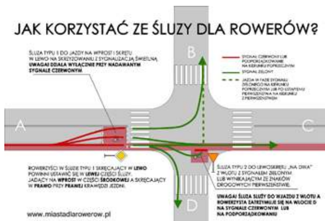
Rysunek 23 Śluzę typu I i II
