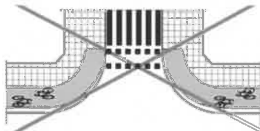
Rysunek 22 Niedopuszczalne odgięcie drogi dla rowerów przed samym przejazdem
