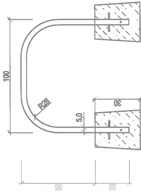
Stojak rowerowy typ "U"
