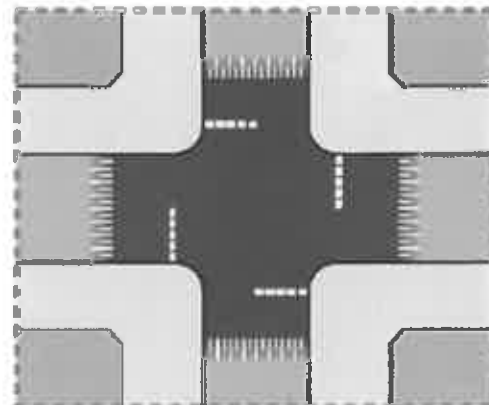
Rysunek 17 Wyniesiona tarcza skrzyżowania
