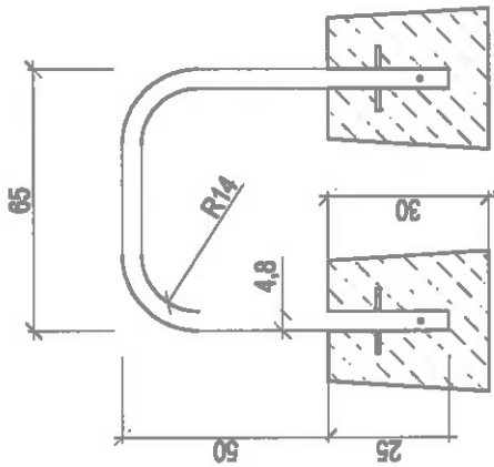
Stojak rowerowy typ "U" mini
